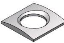
Arruela Diâmetro Ext.: 55,00mm Diâmetro Int.: 32,50mm Espessura: 7,00mm
