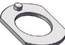
Arruela Diâmetro Ext.: 65,00mm Diâmetro Int.: 36,00mm Espessura: 4,00mm
